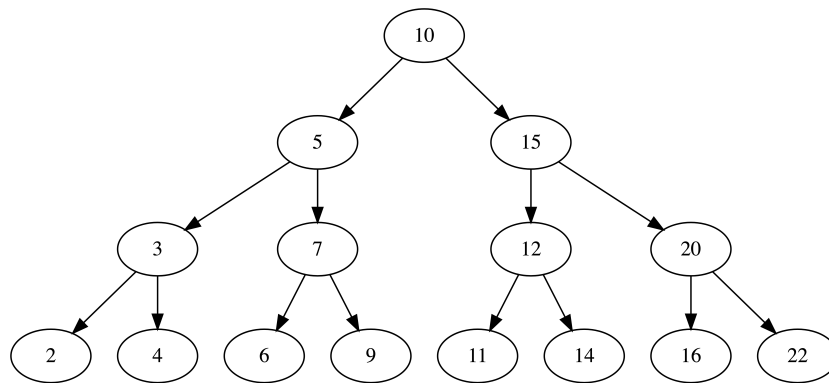
FIGURE 2 – Exemple d'arbre binaire de recherche
